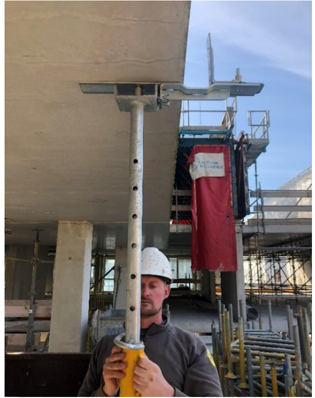
Druk de B-Pro beugel tegen de breedplaat
