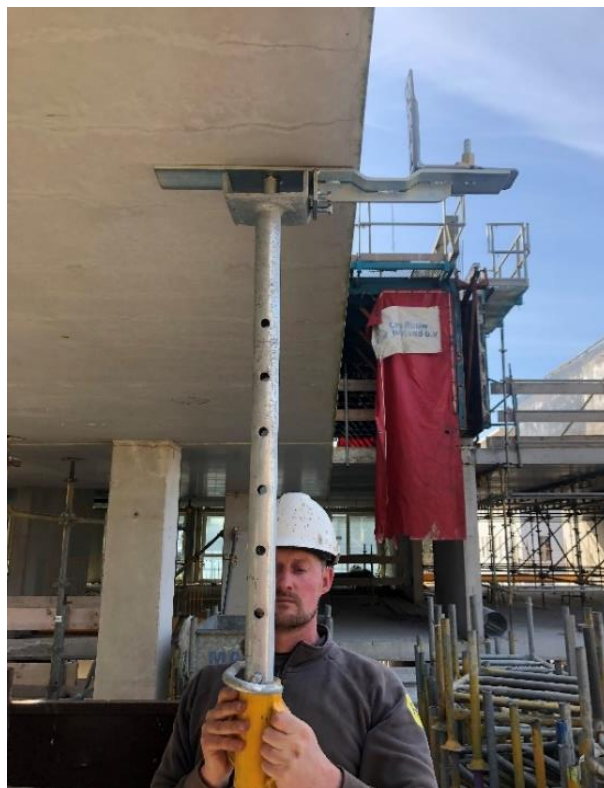
Druk de B-Pro beugel tegen de breedplaat
