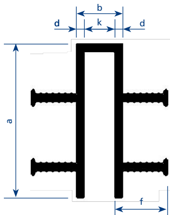
met 4 waterkeringsrillen
