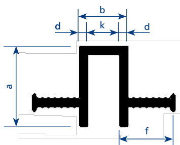
met 2 waterkeringsrillen
