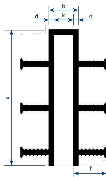
met 6 waterkeringsrillen
