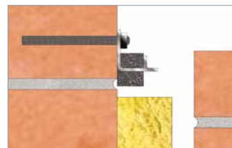
Bevestiging met draadstang M8 + chemische verankering
