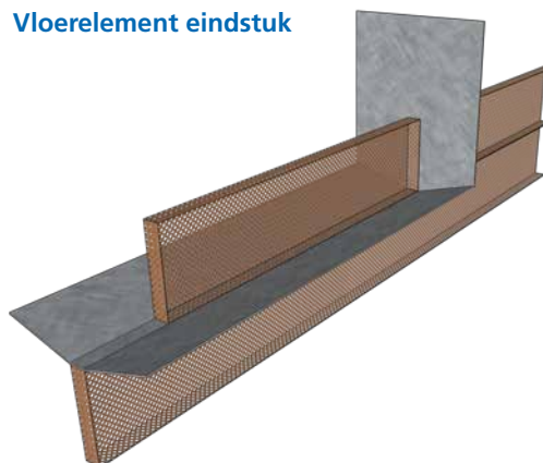
Vloerelement eindstuk
